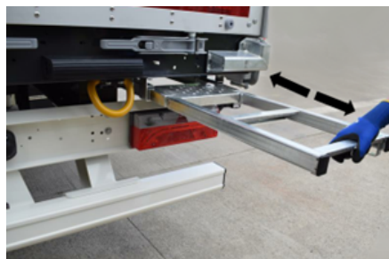
Drabina przesuwno-składana
