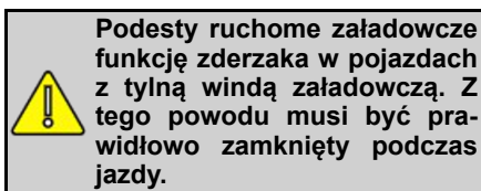
Tylna winda załadowcza typu składanego
